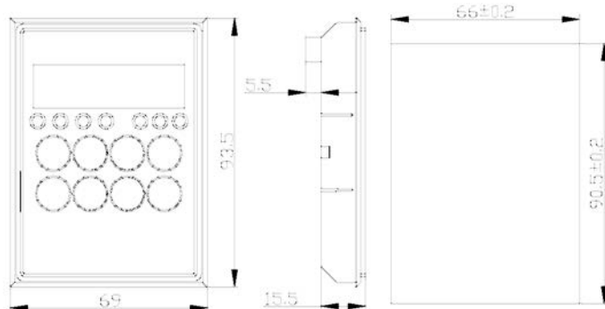
Рис. 3-6. Внешние размеры клавиатуры
