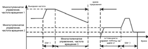
Рис. 6-26 Простой PLC продолжает работать с прерванного шага
