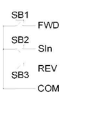
Рис. 6-12. Трехпроводный режим управления 2
