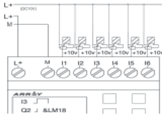
Рис. 2.9 Типы на постоянный ток (DC) D тип
